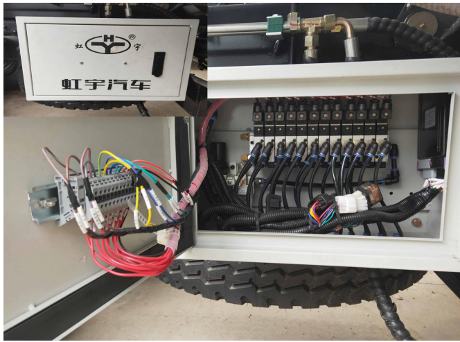
气控箱
